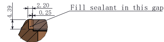
局部视图 B 比例 1 : 1
